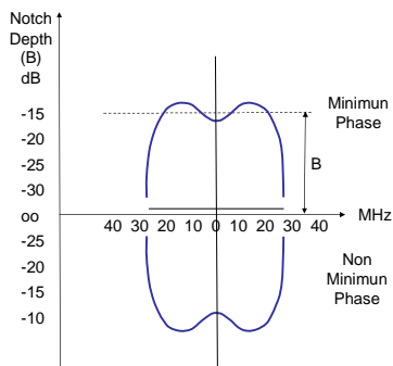
Figura 8.6 Curva Signatura típica
