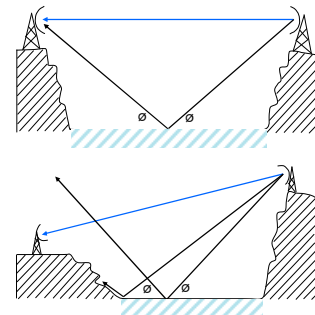
Figura 8.8 Geometría de la Reflexión
