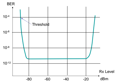
Figura 8.4 BER vs. Nivel de Recepción
